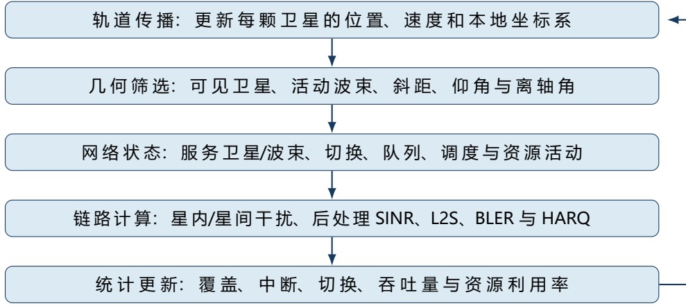
Figure 3: 多卫星系统级仿真的多速率时间循环
